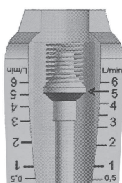
Flödesindikator
