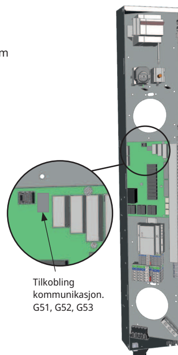
Strømboks EcoZenith
