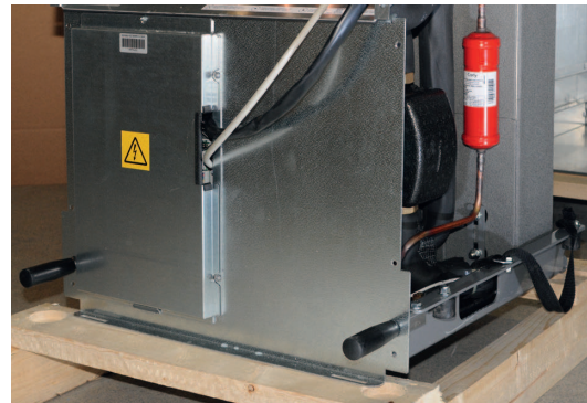
6. Løft kølemodulet ind i produktet ved hjælp af bærehåndtagene og skulderstropperne. Fjern bærehåndtagene, og tilslut ledning, slanger og skruer
