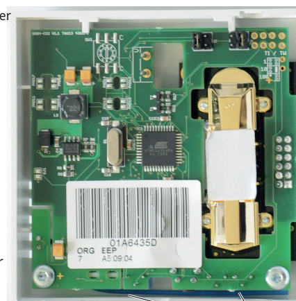
Knop "Leren" (onderaan): om de voeler te verbinden/pairen met de Gateway
