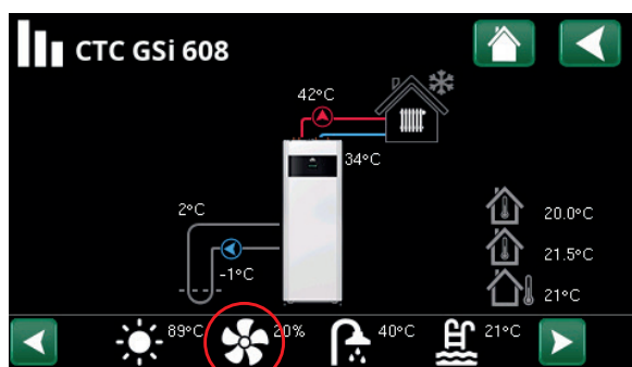
Meny «Driftsinfo»
