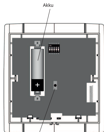
"Learn-painike" anturin perusyksikköön liittämistä tai rinnankytkentää varten
