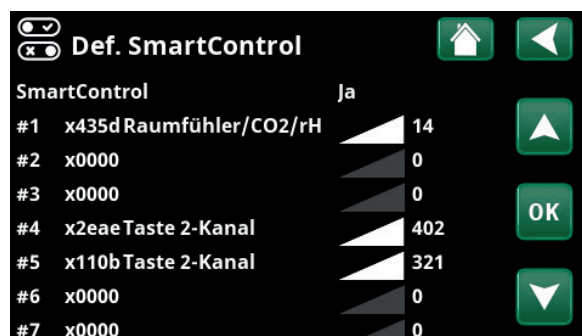
Menü „Fachmann/System/SmartControl“.
