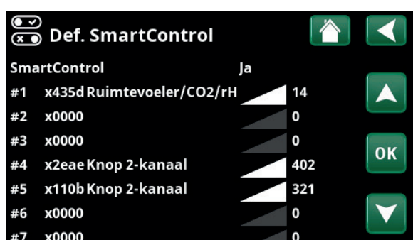
Menu "Installateur/Definieer/SmartControl".
