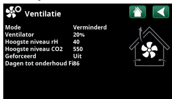
Menu "Werking/Ventilatie".
