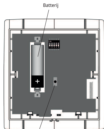
Knop "Leren": om de voeler te verbinden/pairen met de Gateway
