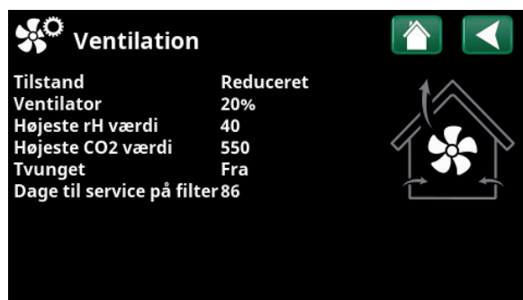
Menu "Driftsinfo/Ventilation".
