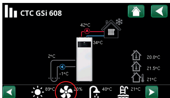
Menü „Betrieb“.
