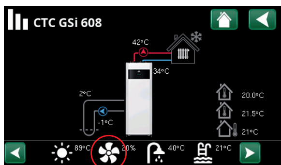
Menu "Driftsinfo".
