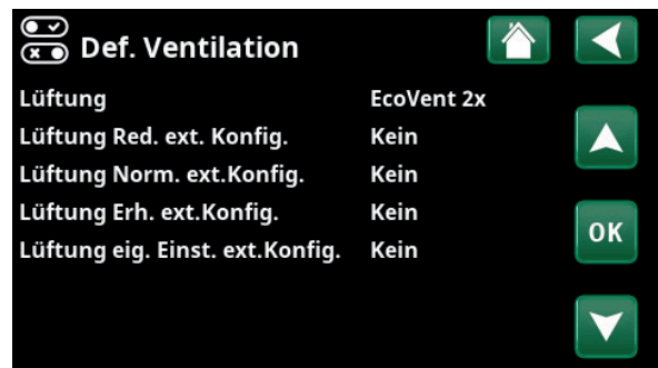
Menü „Fachmann/System/Ventilation“.
