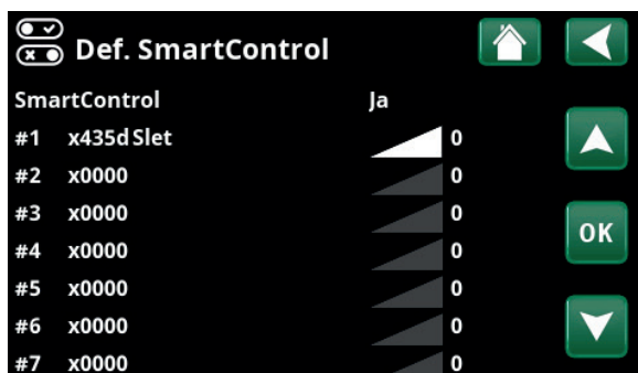
Menu "Avanceret/Definere/SmartControl".
