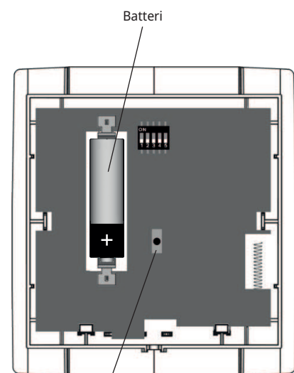
«Learn»-knapp for å koble til / pare føleren med gateway
