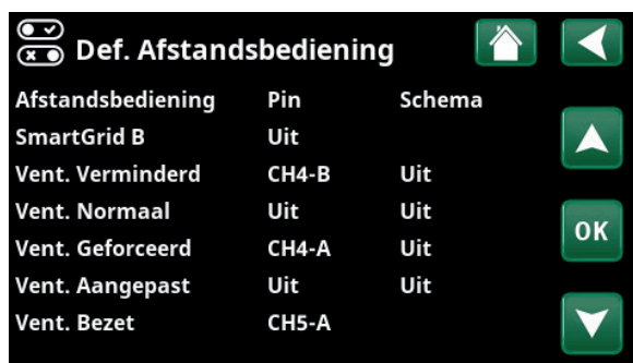
Menu "Installateur/Definieer/Afstandsbediening".
