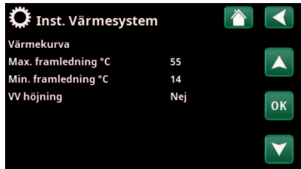
Meny "Avancerat/Inställningar/Värmesystem.
