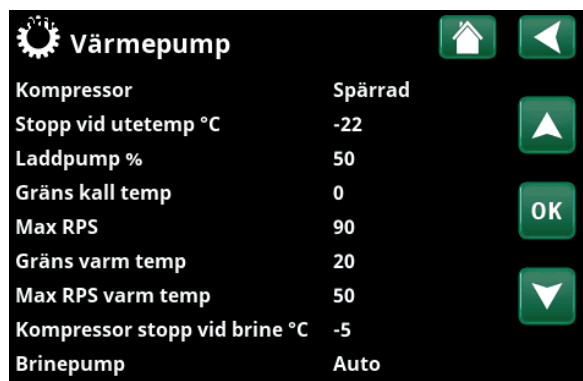
Meny "Avancerat/Inställningar/Värmepump".
