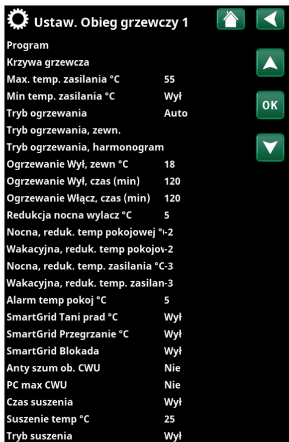
Menü „Instalator\Ustawienia\Obieg grzewczy\Obieg grzewczy 1”.
